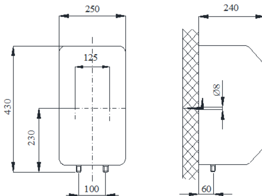
Tehnički crtež
